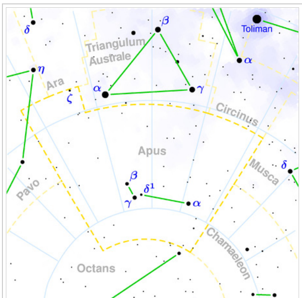
كوكبة طائر الفردوس / Apus
